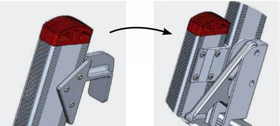
Funcionamento do sistema de fixação do degrau
